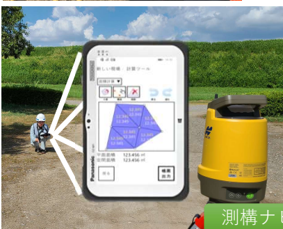
レーザースキャナ
